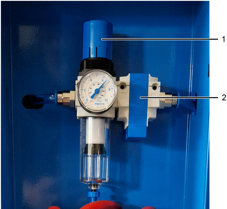
Abb. 34. Manometer
