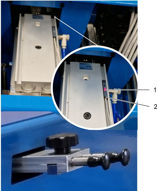
Abb. 40. Linearantrieb
