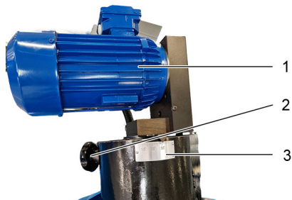
Abb. 3. Schleifsäule
