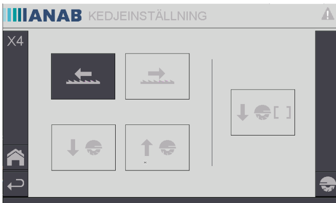
Figure 21. Réglage de la chaîne, étape 1
