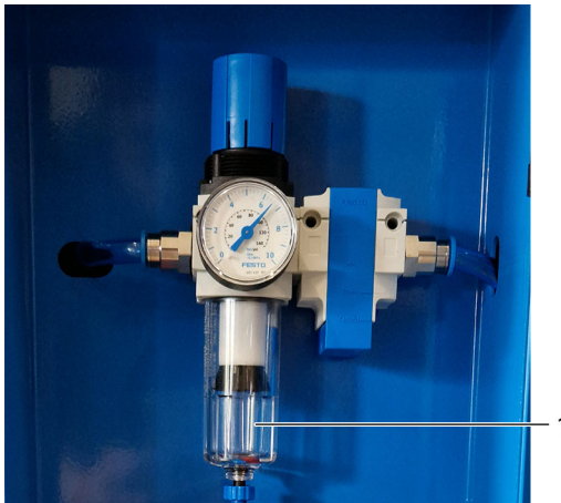
Figure 38. Réservoir en verre avec filtre
