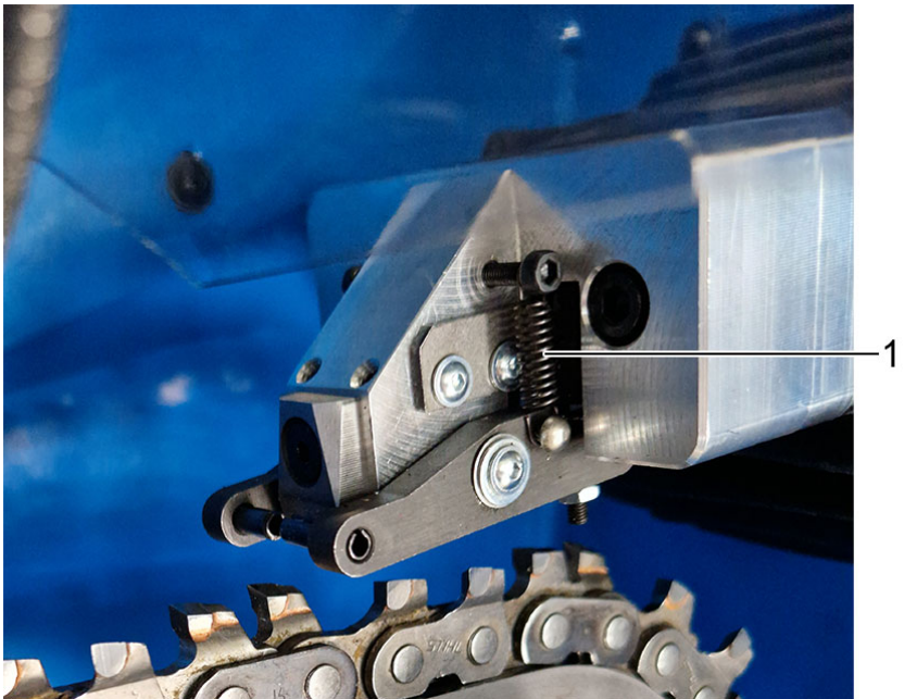
Abb. 42. Mikroschalter am Fühlerfinger
