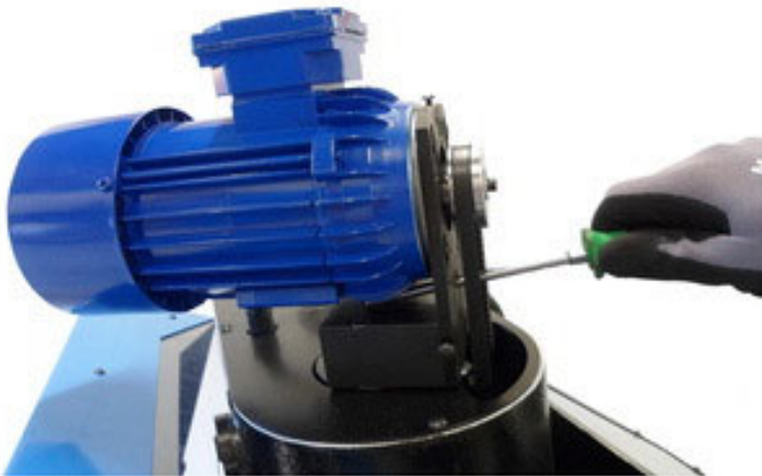
Abb. 45. Riemenspannung
