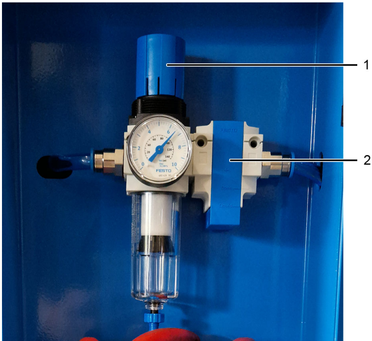
Abb. 40. Manometer
