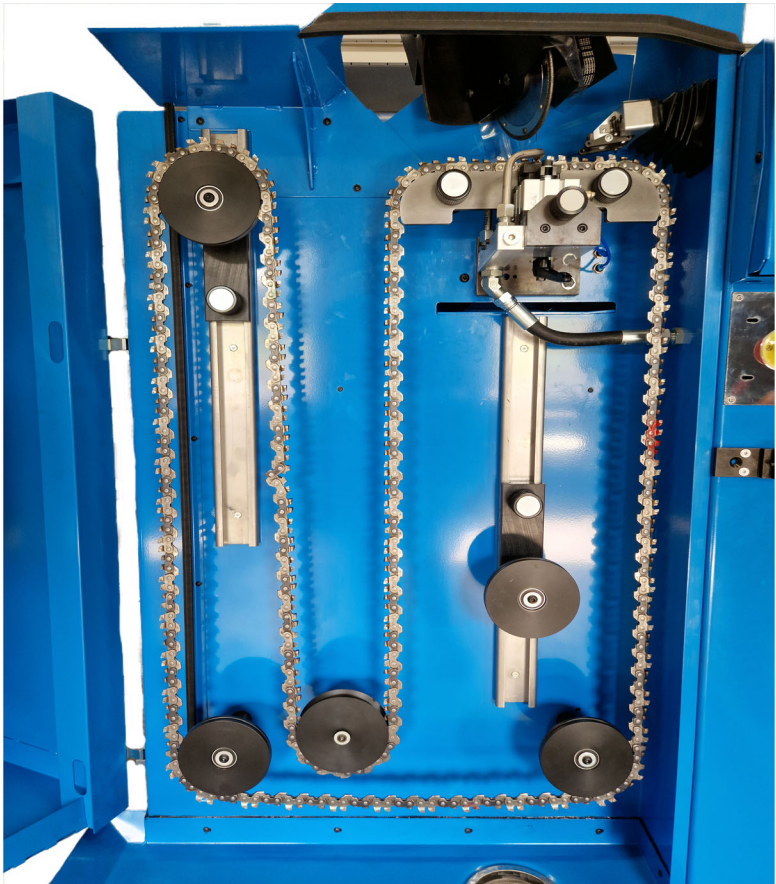
Abb. 50. Kettenhalter, lange Ketten
