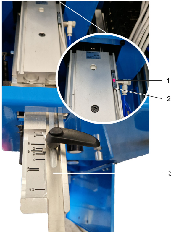
Abb. 46. Linearantrieb
