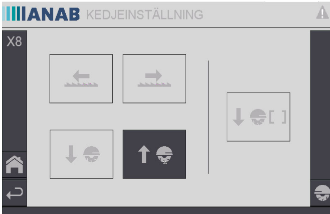
Figure 25. Réglage de la chaîne, étape 4
