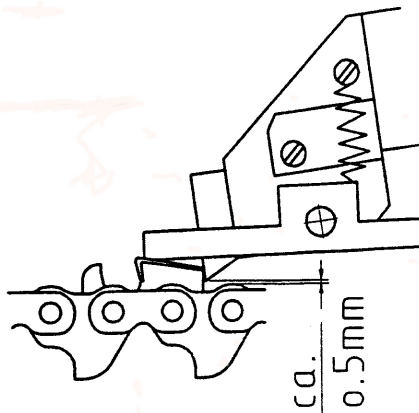
Figure 12. Réglage de la distance
