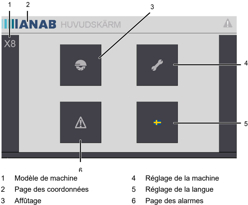
Figure 13. Écran principal tactile
