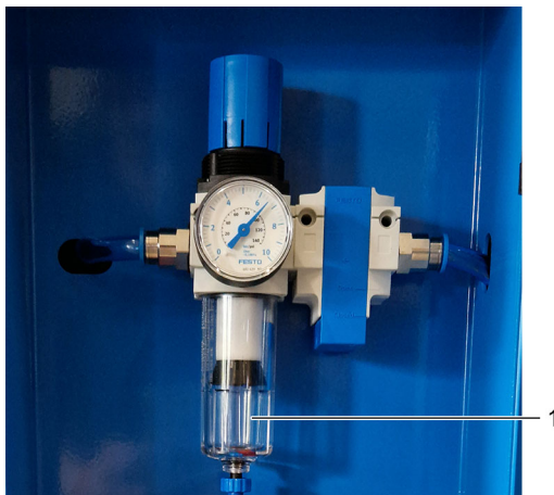
Figure 39. Réservoir en verre avec filtre
